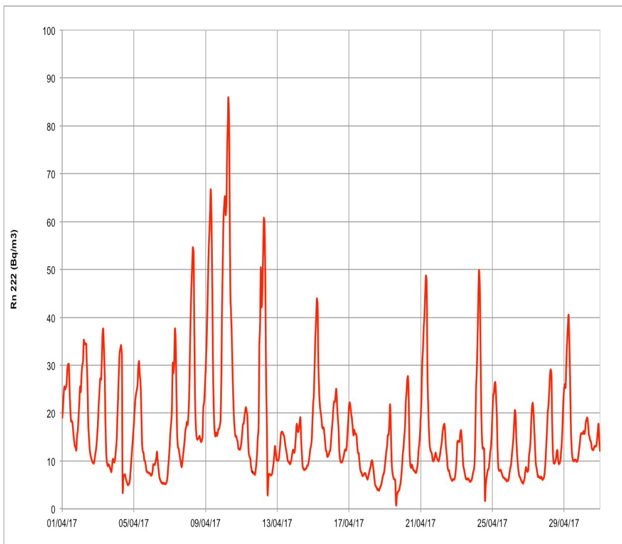
Variations des activités volumiques du radon dans l'air à Luxembourg-Ville.
